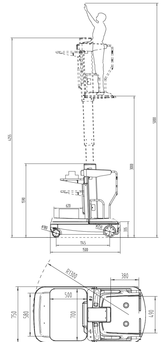
OPSM Dimensions
